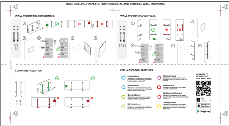
Plantilla para perforar agujeros en la pared
