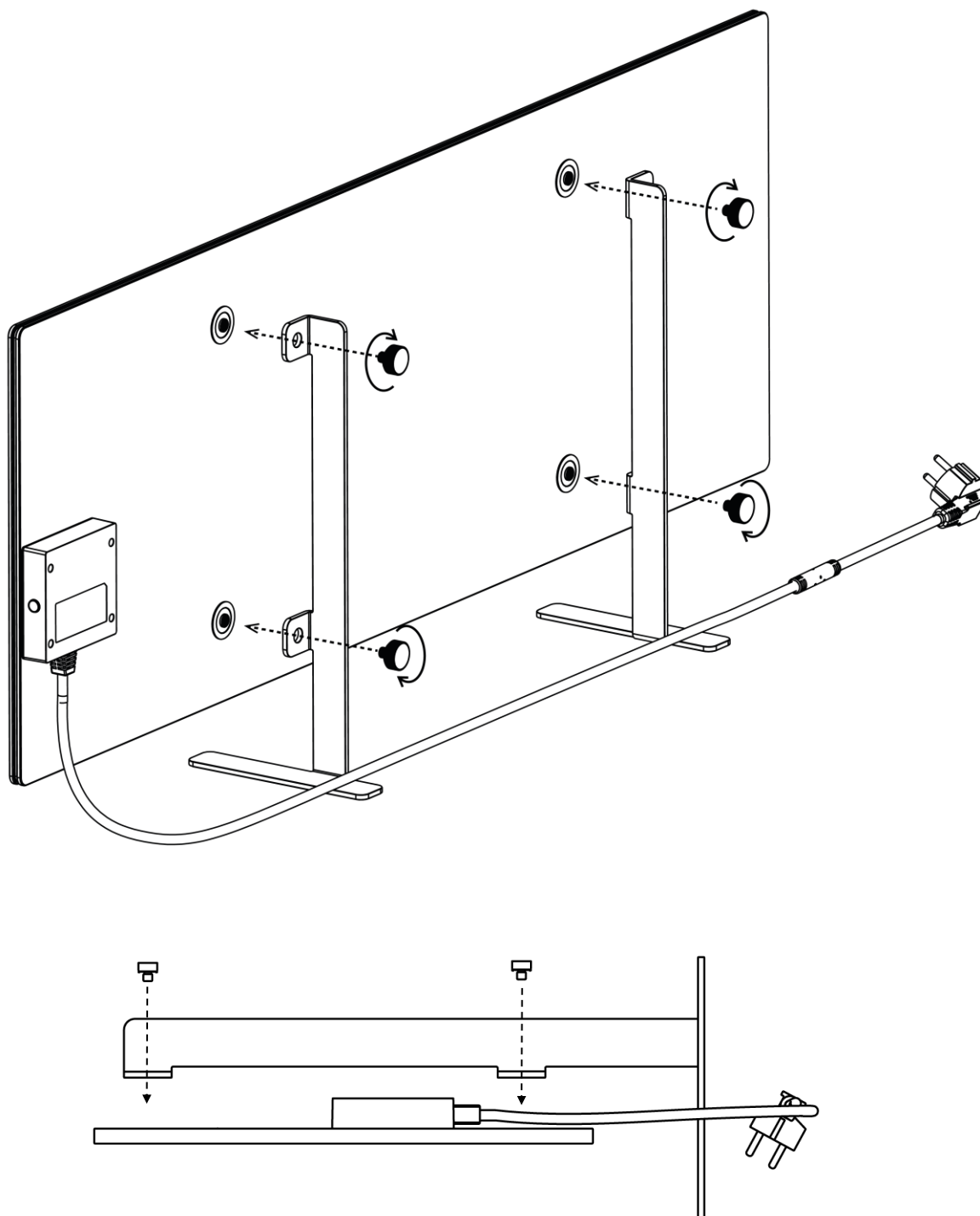
Figura 6 – Montaje en patas (en el suelo)
