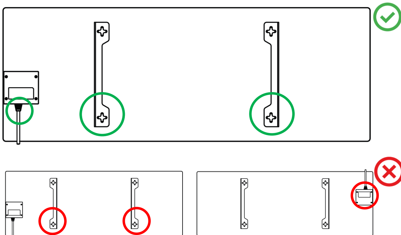
Figura 7 – Instalación de los soportes
