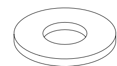
H2 (x4) Ø5x1
