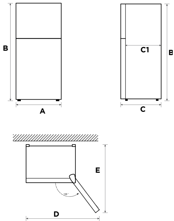
Platzbedarfsdiagramm (bei geöffneter und geschlossener Tür)
