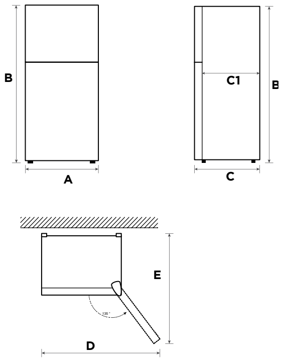
Diagrama de necesidades de espacio (con la puerta abierta y con la puerta cerrada)
