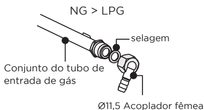
Cotovelo
