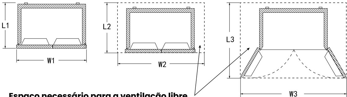
Espaço necessário para a ventilação livre
